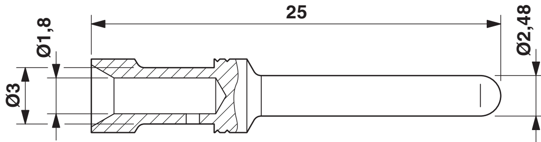
Maßzeichnung
